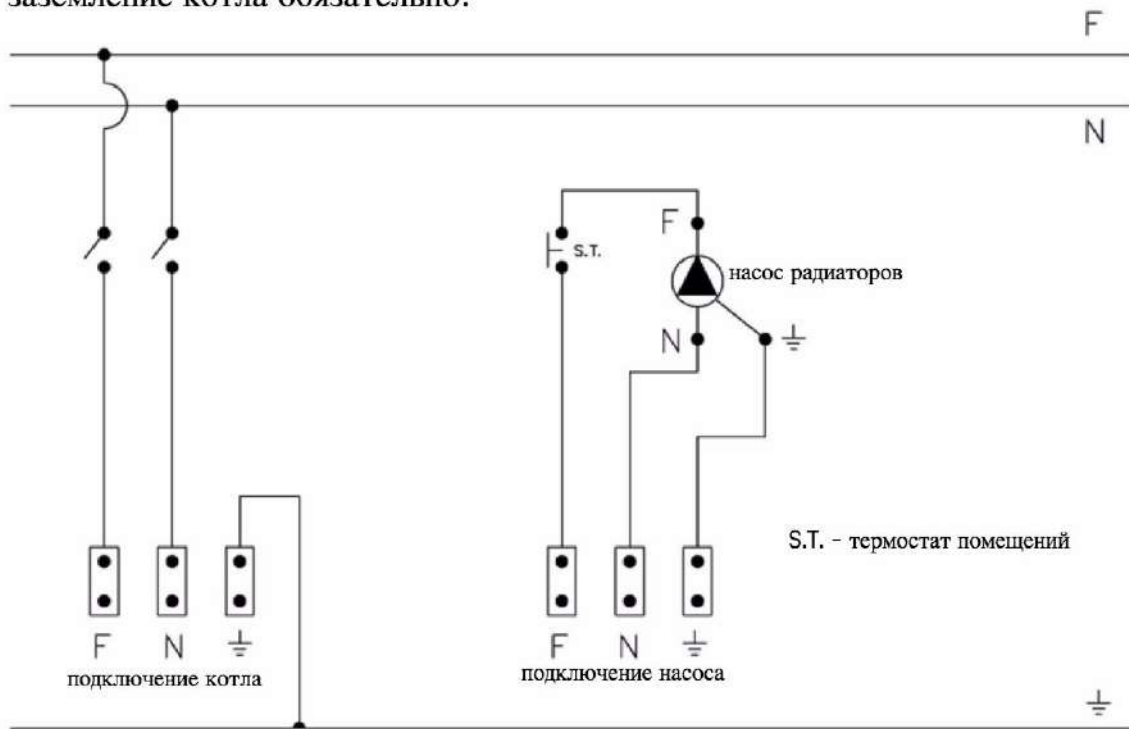
электрическая схема 1
