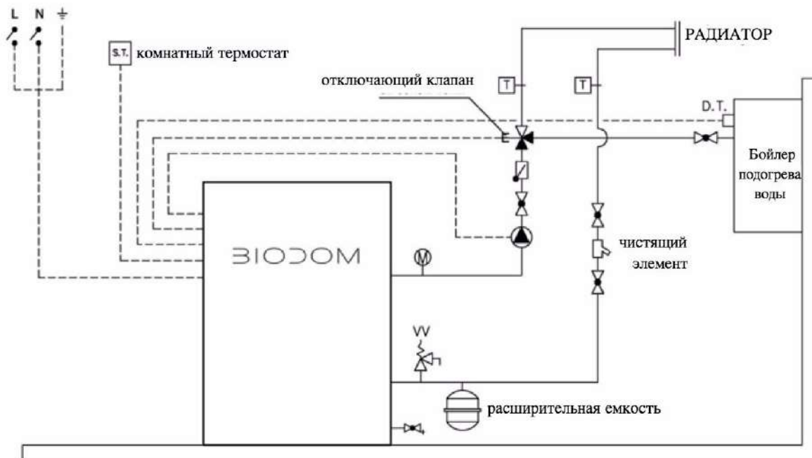
Схема подключения 2
