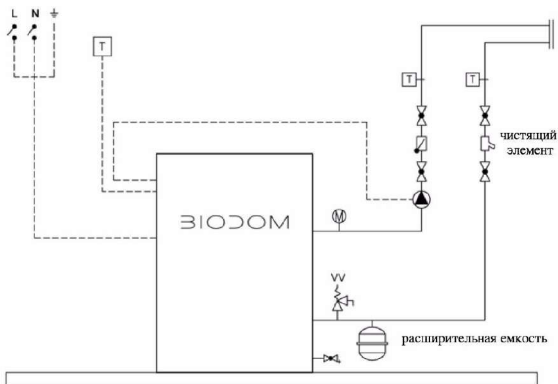
Схема подключения 1
