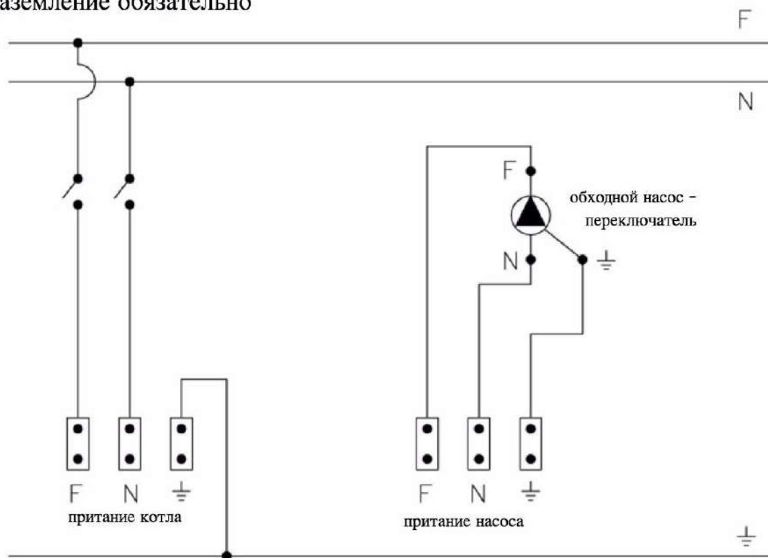
Электрическая схема 3
