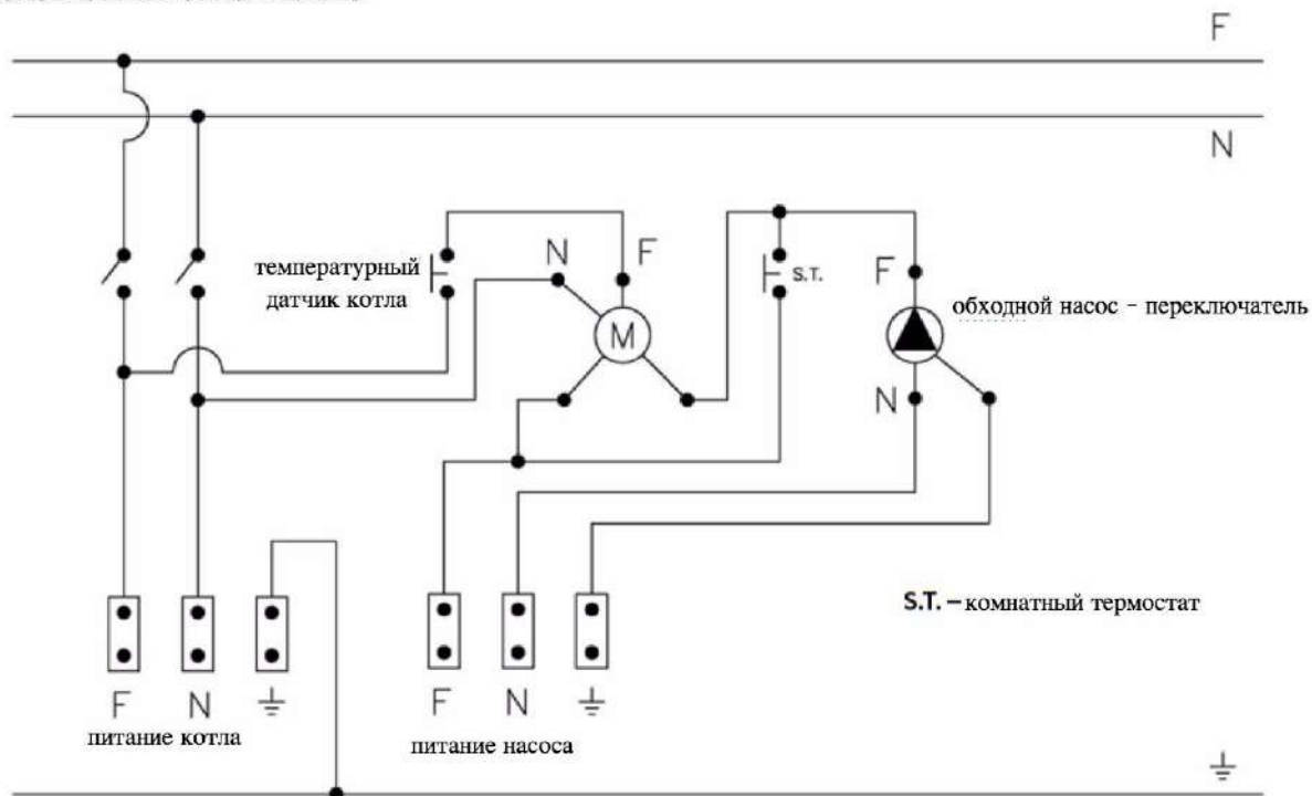
Электрическая схема 2
