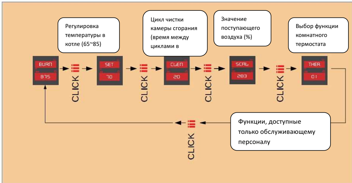
рис. 13: описание меню
