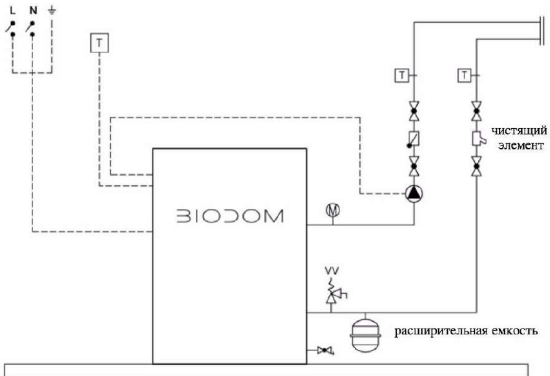
Схема подключения 1
