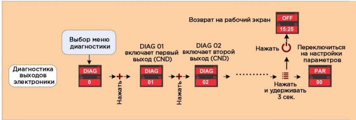
рис. 13: описание меню
