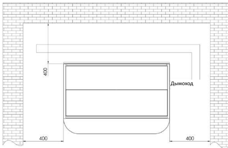
Рис. 1: Минимальное расстояние между котлом и стенами котельной
