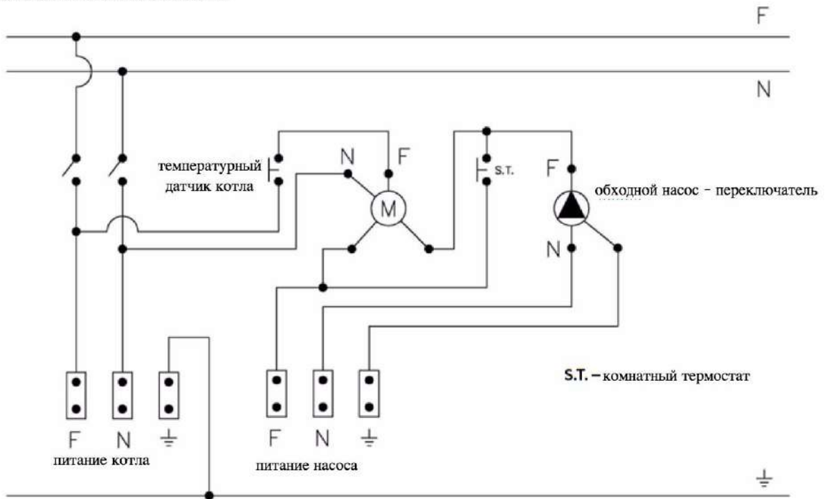
Электрическая схема 2
