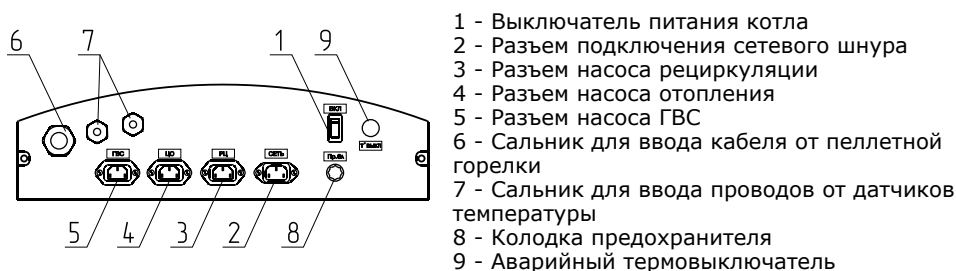
Рис.6. Расположение органов управления на задней панели пульта.
