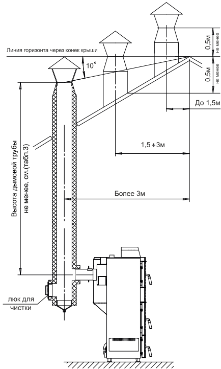
Рис.8. Варианты установки дымовой трубы.
