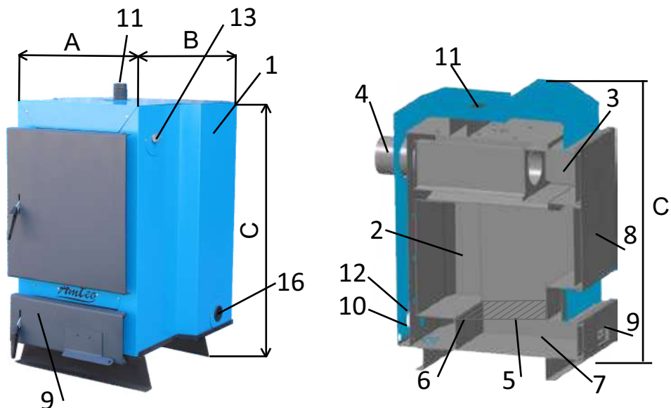
Рис. 1 Котёл «AMTEO»
