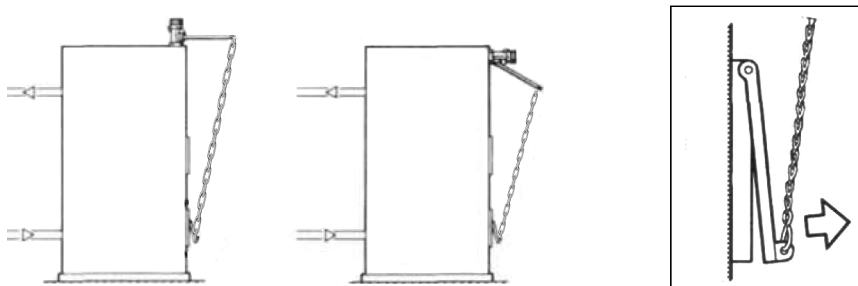
Рисунок 9 – Схема закрепления цепи тягорегулятора на заслонке нижней дверцы котла
